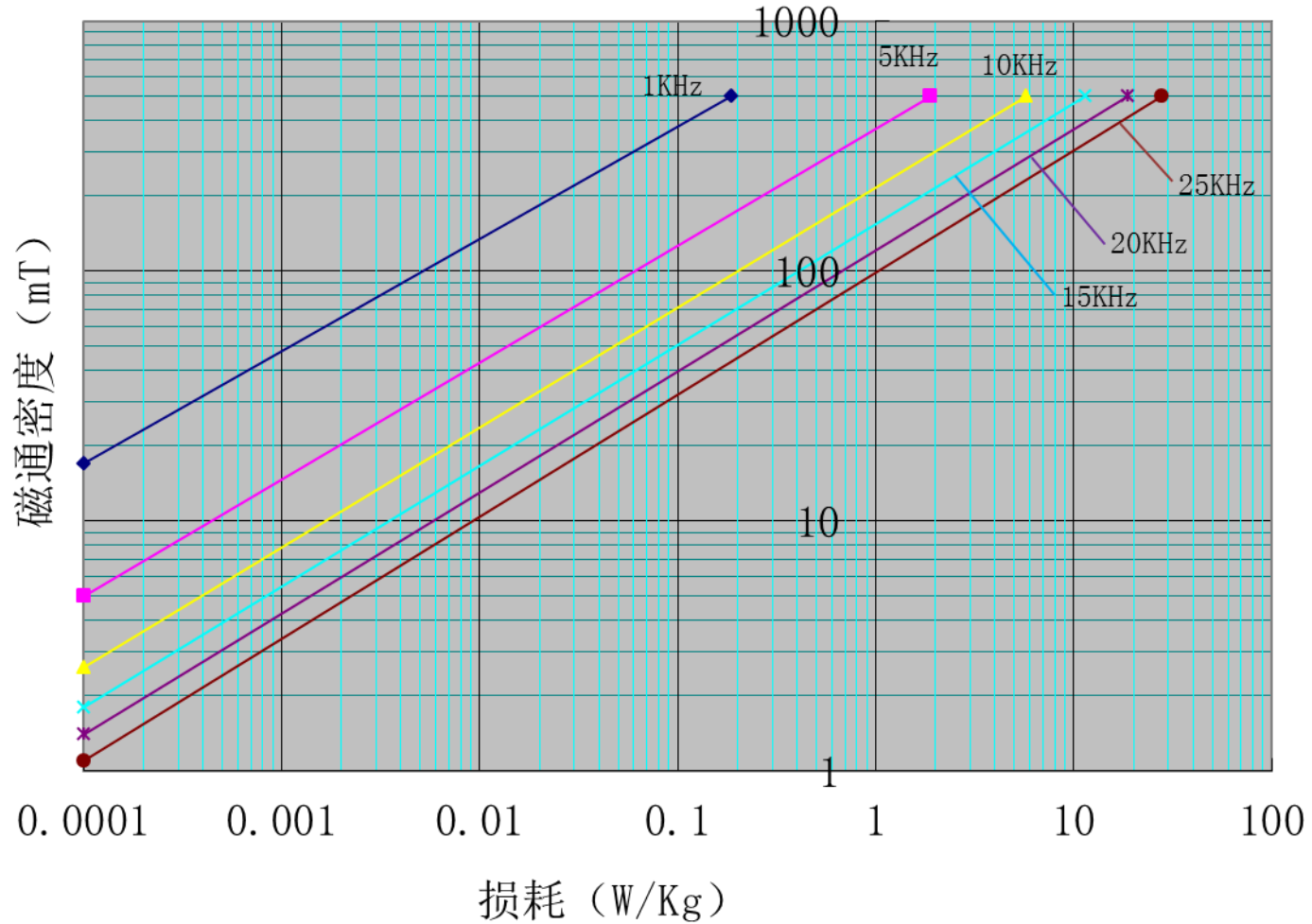
YN-NT-T-805025功率性变压器磁芯不同频率下磁通密度与损耗曲线
